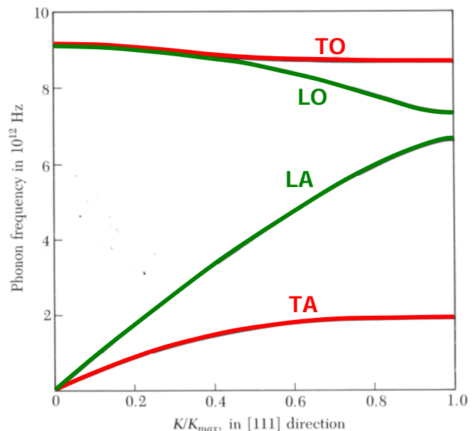
Dispersion für Germanium (80 K) in [111]-Richtung
