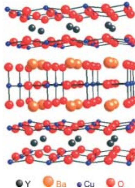
Kristallstruktur eines Hochtemperatur-Supraleiters mit leitenden Schichten (oben und unten).
