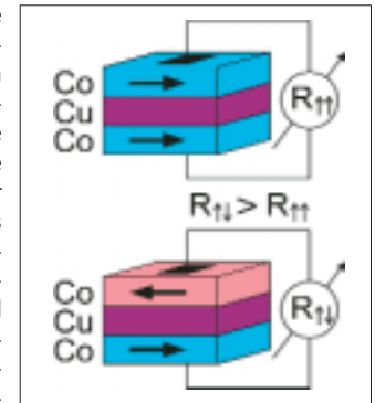
Schichtsystem aus magnetischem und nichtmagnetischem Material. Die Dicke der Zwischenschicht bestimmt die Orientierung der Magnetisierung – und daran gekoppelt den Widerstand.
