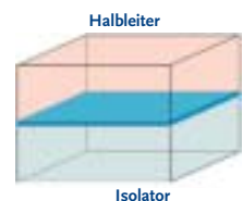
Elektronen an einer ebenen Grenzfläche.
