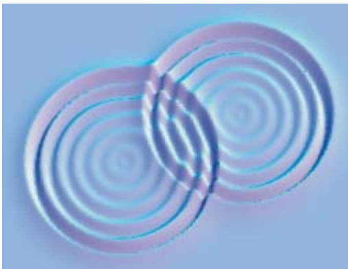
Interferenzmuster bei der Überlagerung zweier kreisförmiger Wellenzüge.
