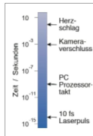
Wie schnell verlaufen verschiedene Prozesse?
