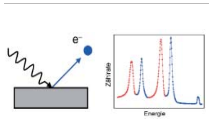
Herauslösung von Elektronen aus einem festen Körper durch Licht (Photoemission): Schema und Resultat für Ytterbium. Rot: Beitrag der Oberfläche.
