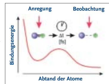
Prinzip der experimentellen Beobachtung des Ablaufs extrem schneller Reaktionen.
