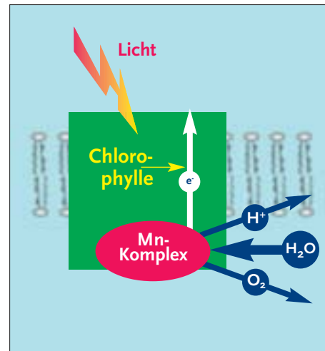
Schema des wasserspaltenen Prozesses am Mangancluster.
