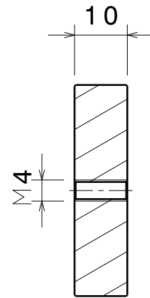
Schnitt A-A
