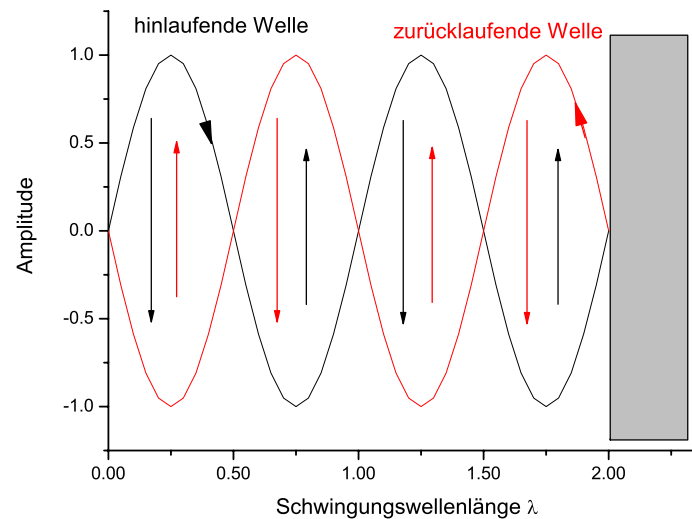
Abbildung 0.18. Interferenzerscheinung der stehenden Welle
