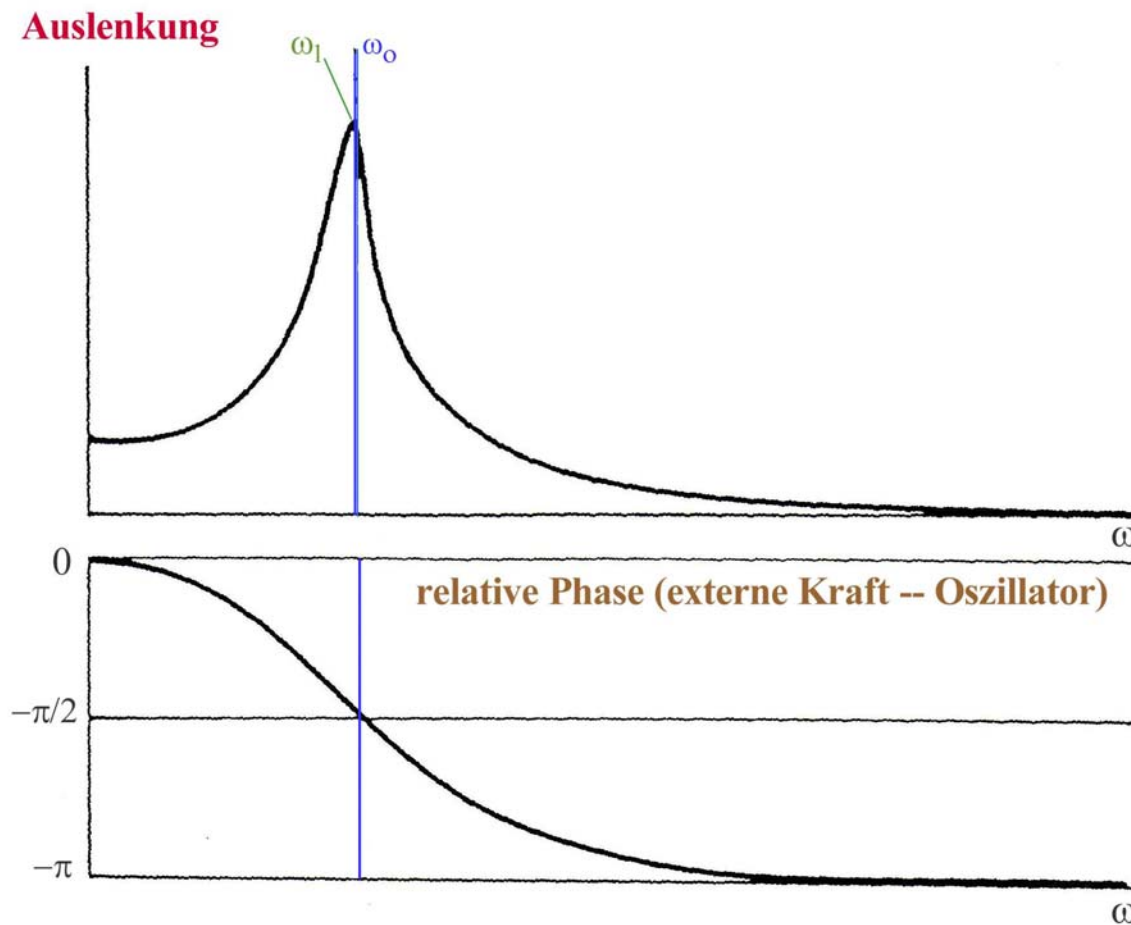
Abbildung 0.13. Die Auslenkung (Amplitude) und die relative Phase eines erzwungenen Oszillators im stationären Zustand als Funktion der externen Frequenz. Bei niedrigen Frequenzen »geht der Oszillator mit«, seine Auslenkung ist genauso groß, wie die Amplitude der externen Kraftquelle. Wenn die externe Frequenz gleich die Eigenfrequenz des Oszillators ist ( \omega_0/\omega_{\text{ext}} = 1 ), ist die Leistungsübertragung optimal, es gibt eine »Resonanzüberhöhung« der Auslenkung. Die maximale Auslenkung findet man jedoch bei der gedämpften Frequenz, \omega_{\text{ext}} = \omega_1 . Steigt die externe Frequenz noch weiter, so nimmt die Auslenkung wieder ab und geht gegen Null für hohe Frequenzen. Die relative Phase zwischen externer Kraftquelle und Oszillator ist Null für kleine Frequenzen, 90^\circ bei Resonanz, und geht gegen 180^\circ für große externe Frequenzen.
