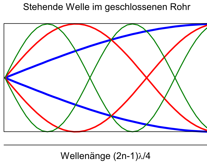
Abbildung 0.19. Stehenden Welle im einseitig geschlossenen Rohr
