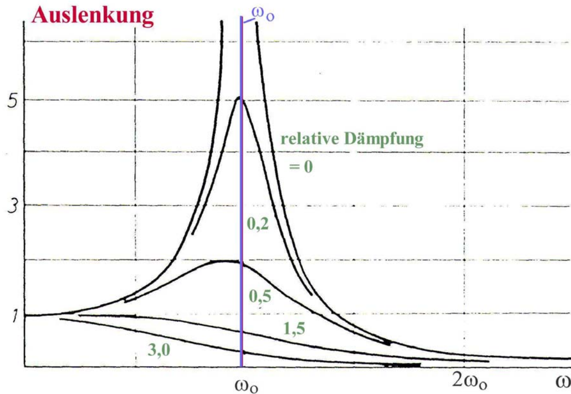
Abbildung 0.14. Die Auslenkung eines erzwungenen Oszillators der Eigenfrequenz \omega_0 in Abhängigkeit der externen Frequenz \omega für verschiedene relative Dämpfungsfaktoren k/\sqrt{mD} . Bei kleiner Dämpfung wächst die Auslenkung im Resonanzfall gegen Unendlich (Resonanzkatastrophe!). Bei großer Dämpfung gibt es keine Resonanzüberhöhung der Auslenkung mehr. Die Breite der Resonanzkurve wird geringer, wenn die Dämpfung kleiner wird.
